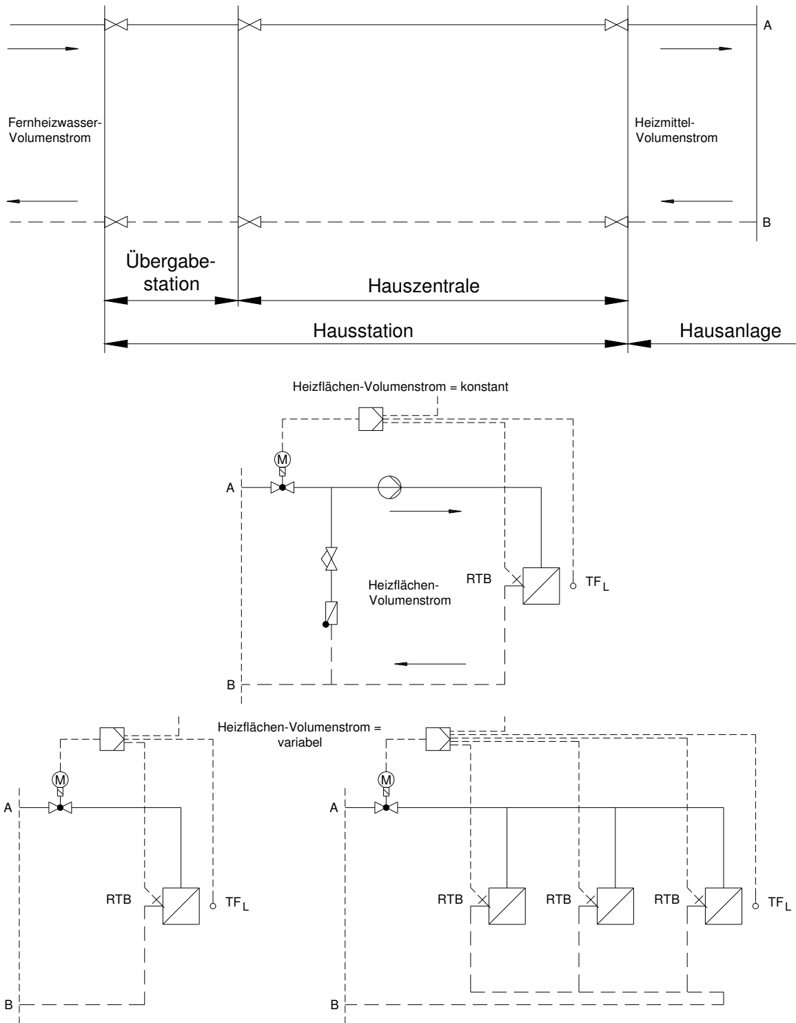
Bild 5: Hauszentrale-Raumluftheizung (RLH)
